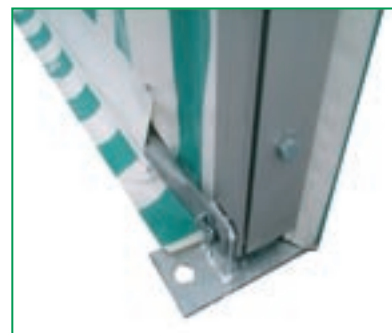
Dettaglio del tensionamento inferiore del telo.
